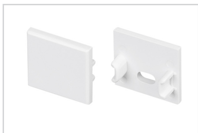
040942 FANTOM-BENT-W16 WHITE
