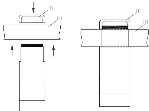
Рис. 2. Установка светильника
